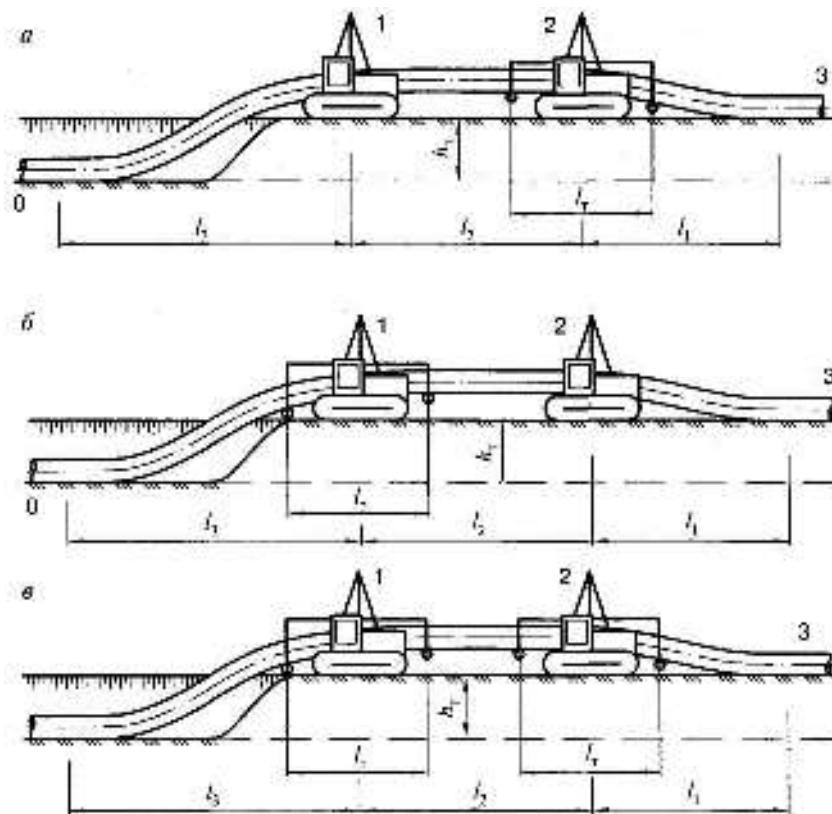
a — с траверсой головного трубоукладчика; б — с траверсой у заднего трубоукладчика; в — с траверсами у обоих трубоукладчиков; 1 — задний трубоукладчик; 2 — головной трубоукладчик; 3 — трубная плетель
