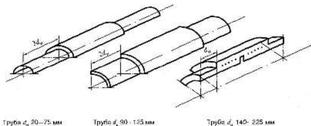
Рисунок Т.1 — Общий вид образцов-сегментов
